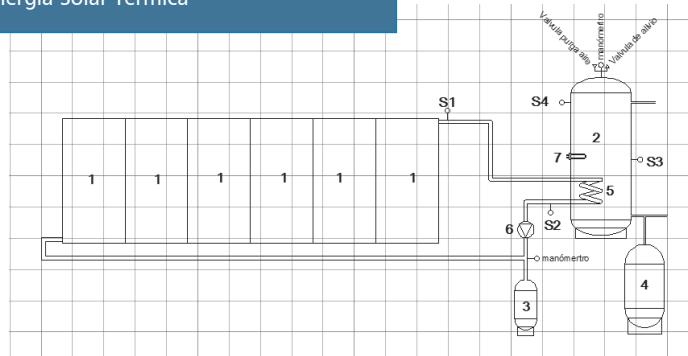
Fig. 01: Diagrama Simplificado del Circuito de Captación y Almacenamiento de Energía Solar Térmica
