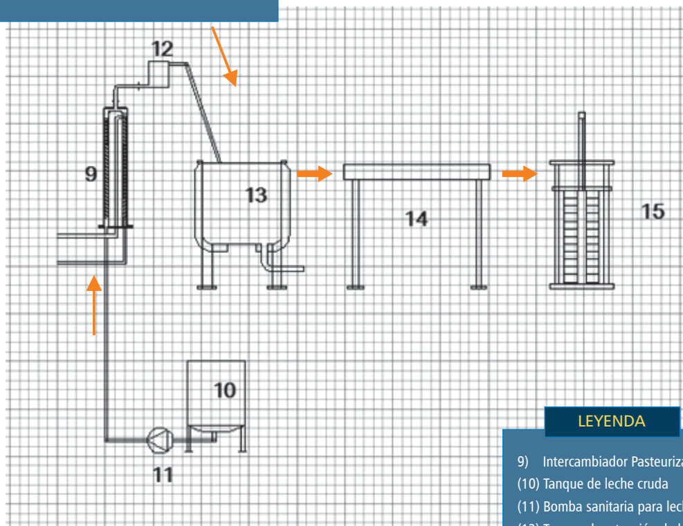
Figura 03: Esquema Simplificado de las instalaciones de la planta de fabricación de derivados lácteos
